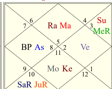
Ghatika Lagna
