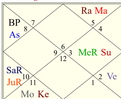
Hora Lagna
